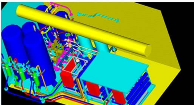
Instalación y Armado del sistema de tuberías Osmosis Inversa BAP. Unión
