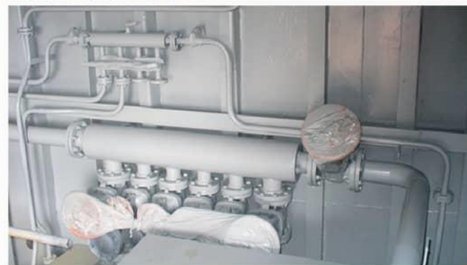
Instalación de tuberías motor principal y otros sistemas – Remolcador BAP Morales
